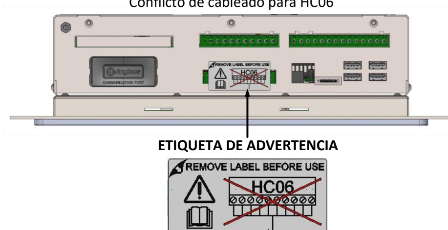
Figura 5: Etiqueta de advertencia de conflicto de cableado del HC06
