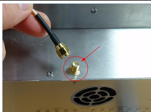
Figura 7: Localización del conector de la antenna wifi
