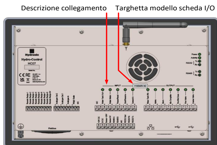
Figura 2: Retro di Hydro-Control – Targhette dei connettori
