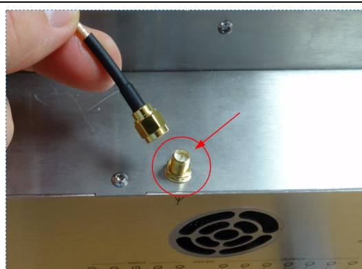
Figura 7: Posizione del connettore dell'antenna Wi-Fi
