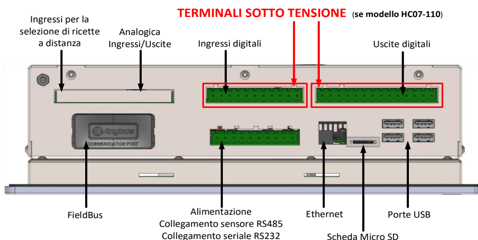
Figura 3: Base del dispositivo Hydro-Control con l'indicazione dei connettori elettrici
