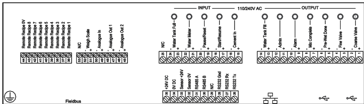
Figura 4: Etichetta descrittiva dei collegamenti elettrici
