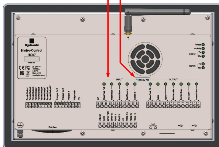
Anschlussbeschreibung E/A-Karten-Modellbezeichnung
