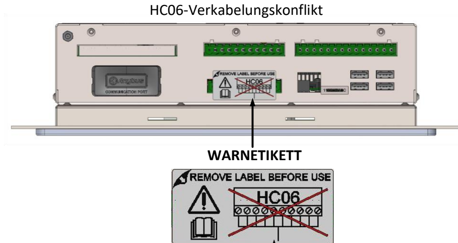
Abbildung 5: Etikett zur Konfliktwarnung bei der HC06-Verkabelung
