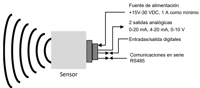
Ilustración 1: Conexión del sensor (descripción general)
