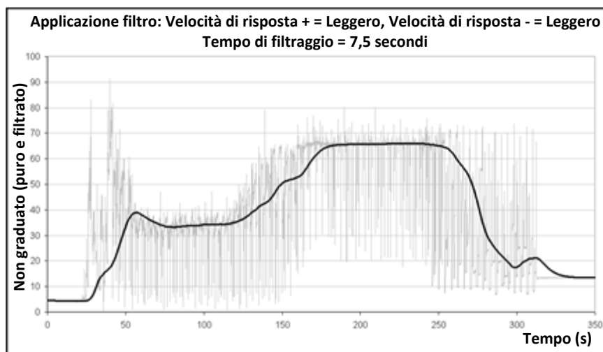
Figura 8. Filtraggio del segnale PURO (2)
