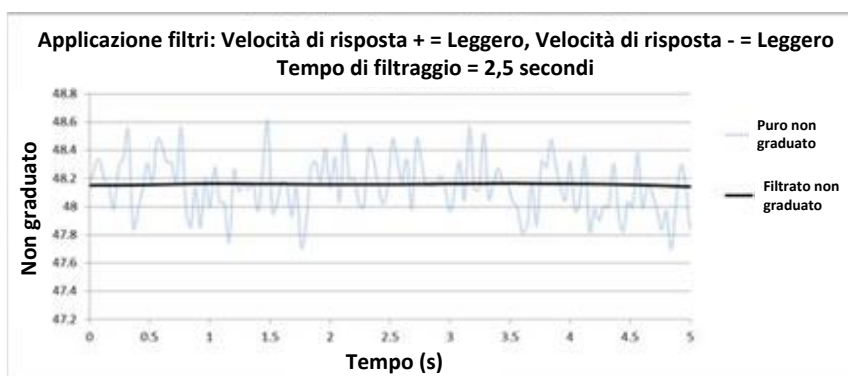
Figura 4. Grafico che mostra il segnale filtrato
