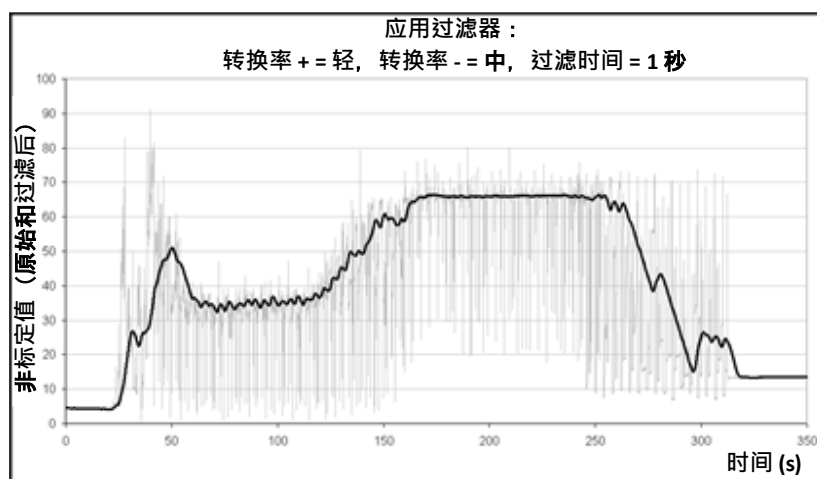
图 7：过滤原始非标定信号 (1)
