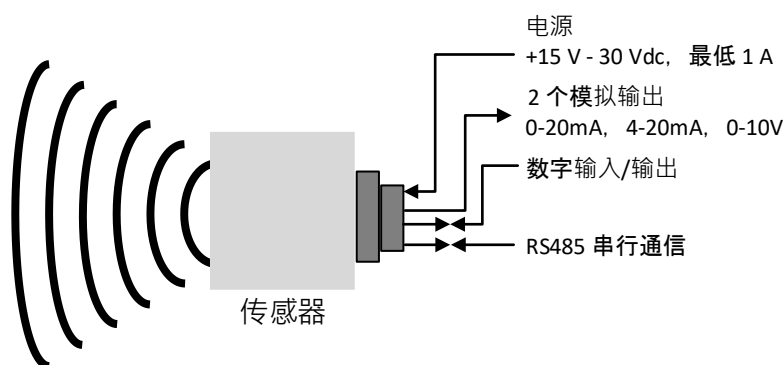
图 1：连接传感器（概述）
