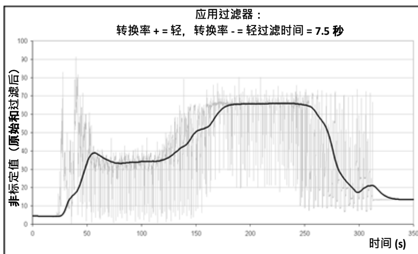
图 8：过滤原始信号 (2)
