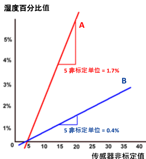
图 9：非标定值和湿度之间的关系
