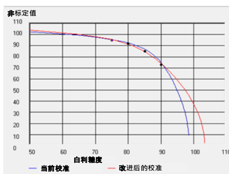
图 21：良好白利糖度校准示例
