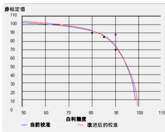
图 22：不良白利糖度校准示例
