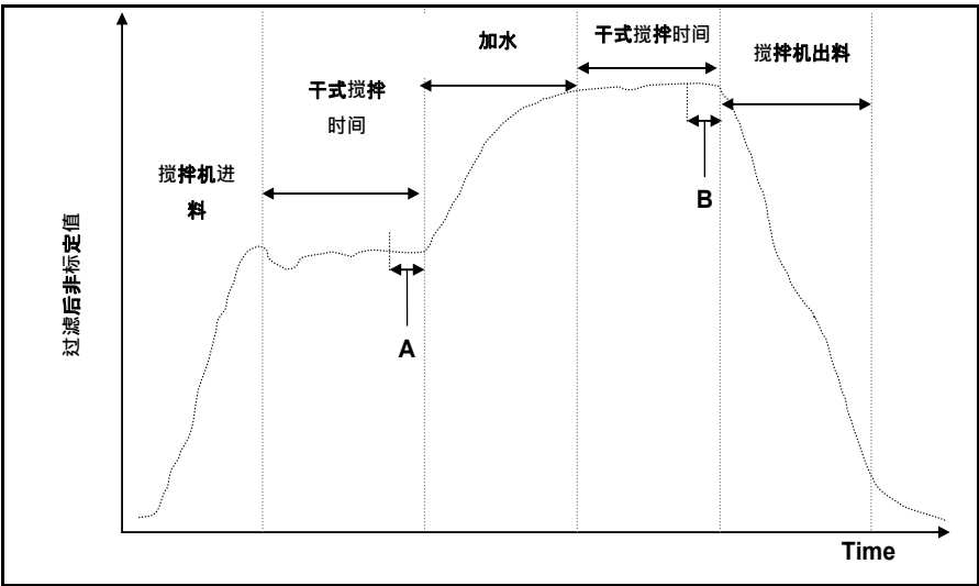
图 5：典型湿度曲线
