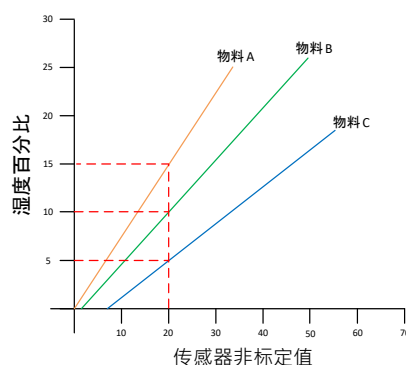
图 13：3 种不同物料的校准
