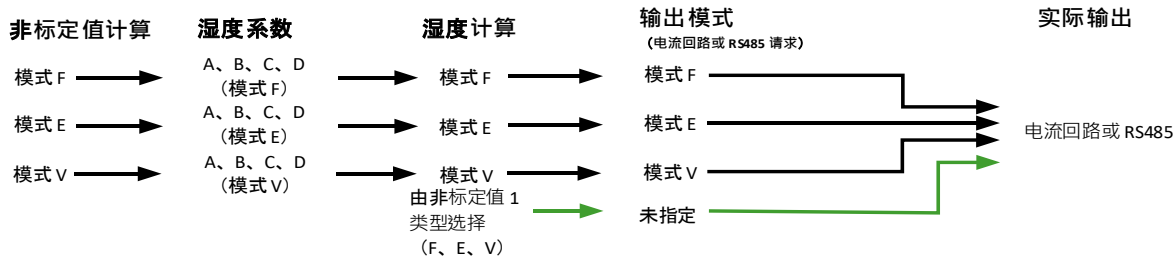
图 11：未指定输出选择
