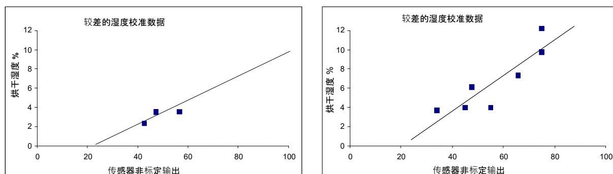
图 18: 较差的物料校准点的示例
