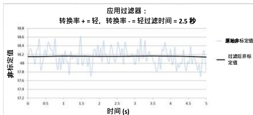
图 4：显示过滤后的信号的图表
