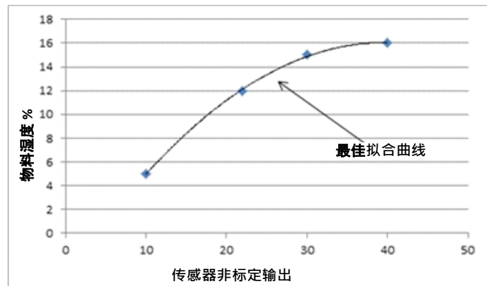
图 19：良好二次校准示例
