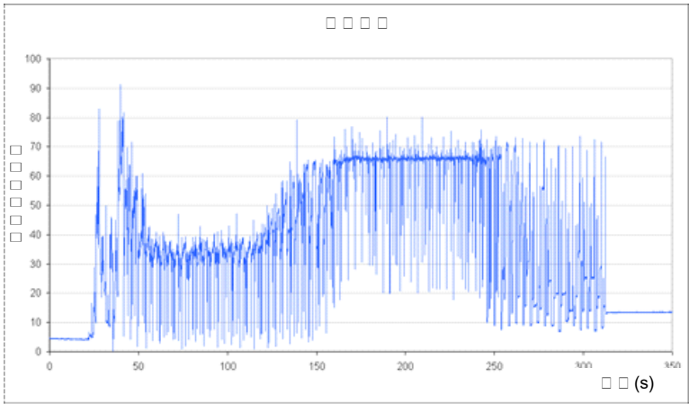
图 6：显示搅拌周期中的原始信号的图表
