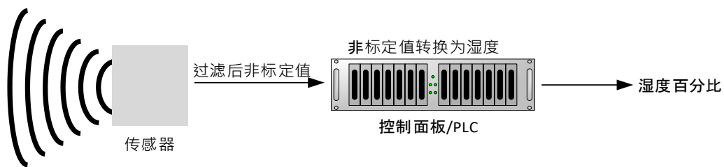
图 16：在控制系统内校准
