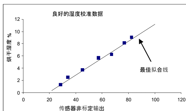
图 17: 良好物料校准示例
