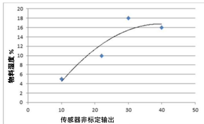
图 20：不良二次校准示例
