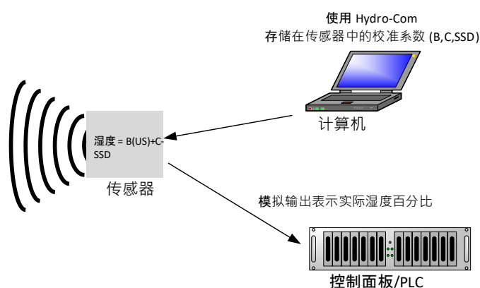
图 15：在传感器内校准
