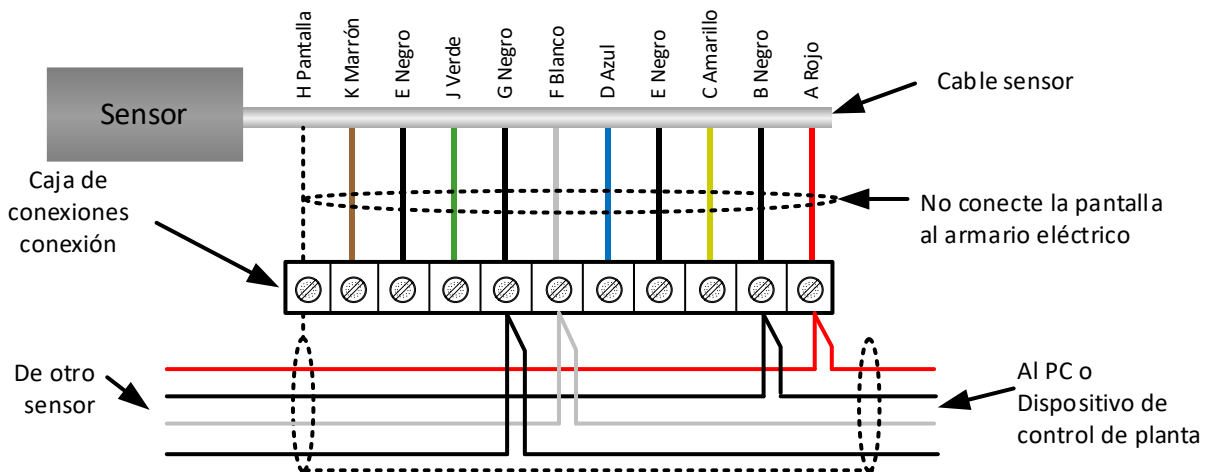
Ilustración 3: Conexiones de multiderivación RS485
