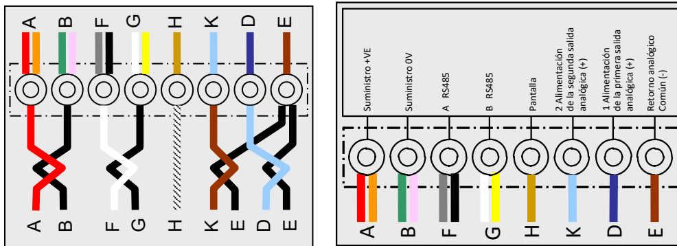
(A) Conexiones del cable del sensor (B) Conexiones de cableado de la planta
