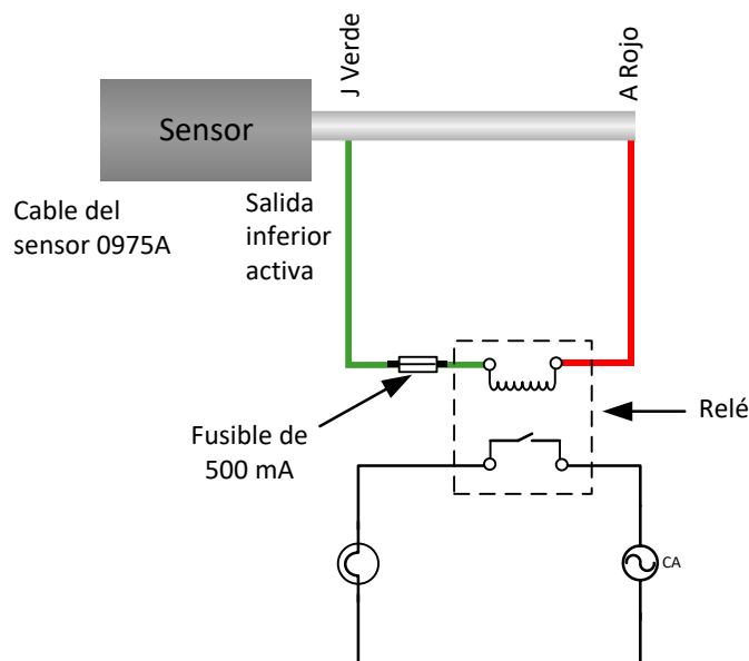
Interruptor de salida digital: ejemplo mediante la utilización de la señal "Cuba vacía" para encender un indicador
