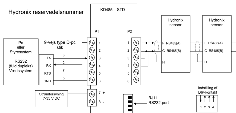
Fig. 12: RS232-RS485-adaptertilslutninger (0049A)
