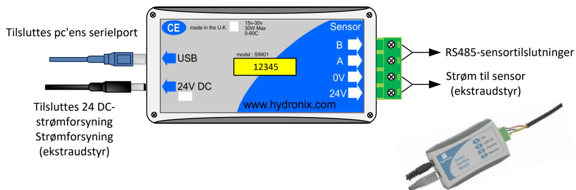
Fig. 13: RS232-RS485-adaptertilslutninger
