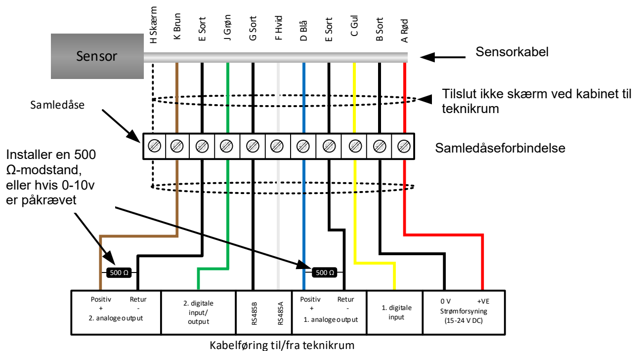
Fig. 1: 0975A-sensorkablets tilslutninger
