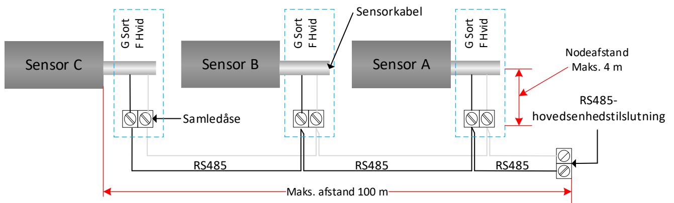
Fig. 2: RS485-multidrop-netværkstopologi
