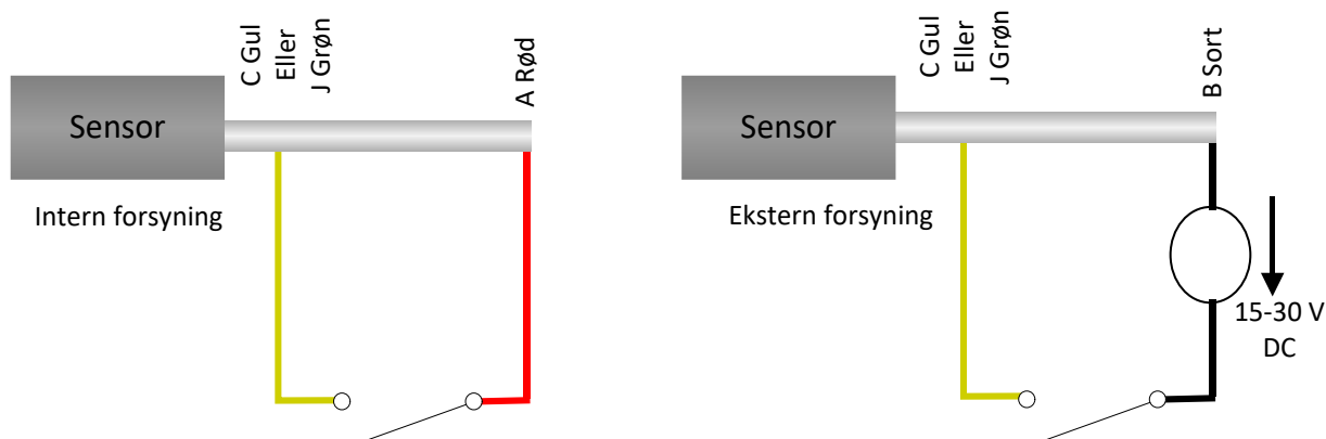
Fig. 6: Intern/ekstern forsyning til digitalt input 1 og 2
