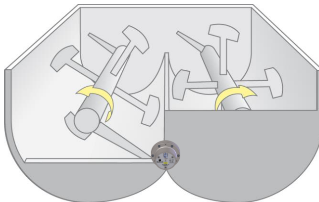
Figura 5: Instalação do misturador de veio duplo orgânico
