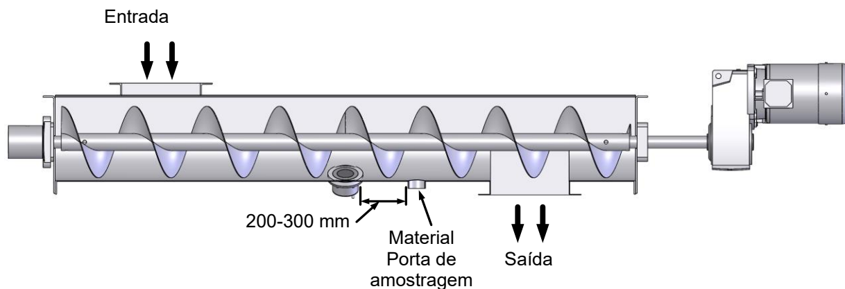
Figura 9: Instalação do transportador helicoidal
