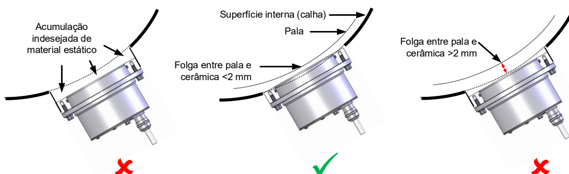
Figura 4: Instalação em superfície curva
