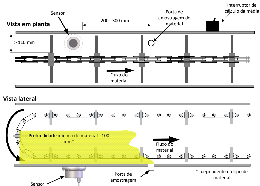
Figura 15: Instalação do transportador de corrente simples
