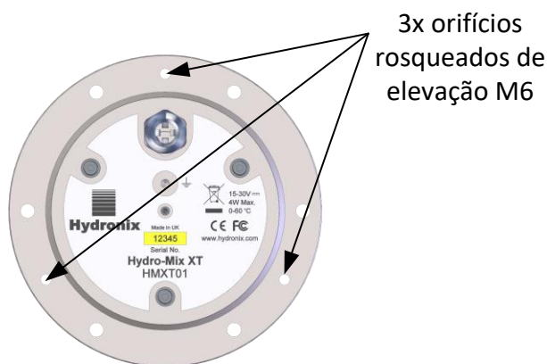
Figura 25: Orifícios de elevação
