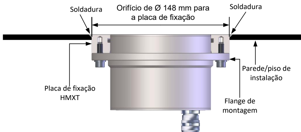
Figure 19: Instalação do sensor (placa de fixação montada à face)
