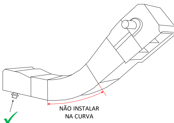
Figure 17: Transportador de corrente inclinada
