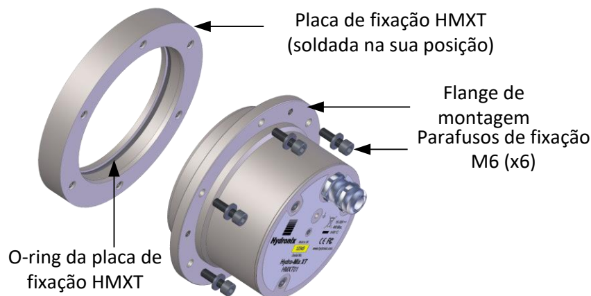
Figura 20: Componentes de montagem do Hydro-Mix XT
