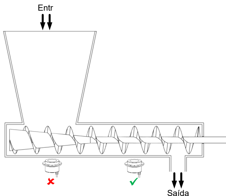
Figura 13: Transportador de fluxo de massa
