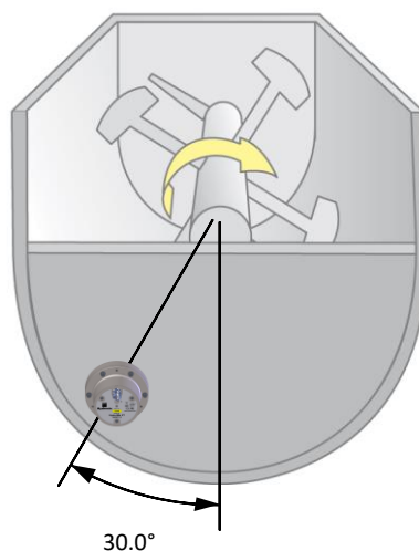
Figura 6: Instalação do misturador de veio simples orgânico
