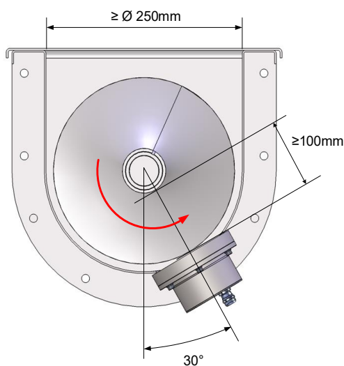
Figura 8: Transportador helicoidal Ângulo de montagem
