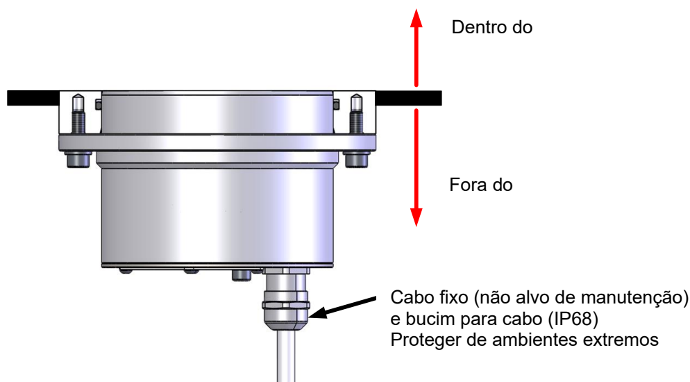
Figure 2: Condições de instalação no exterior
