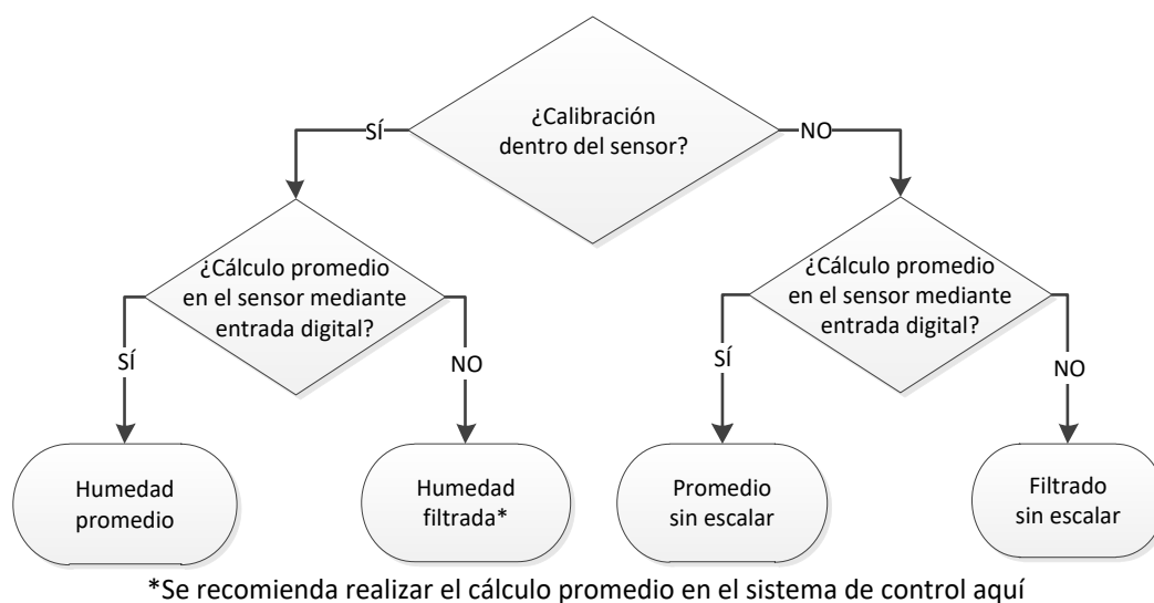
Ilustración 2: Instrucciones para ajustar variables de salida
