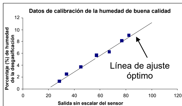
Ilustración 17: ejemplo de una buena calibración del material
