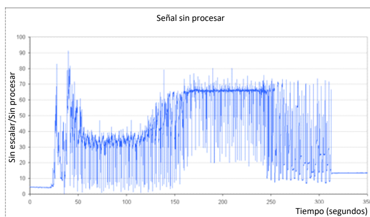
Ilustración 6: Gráfico que muestra la señal sin procesar durante el ciclo de mezcla
