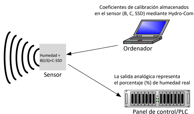
Ilustración 15: Calibración dentro del sensor
