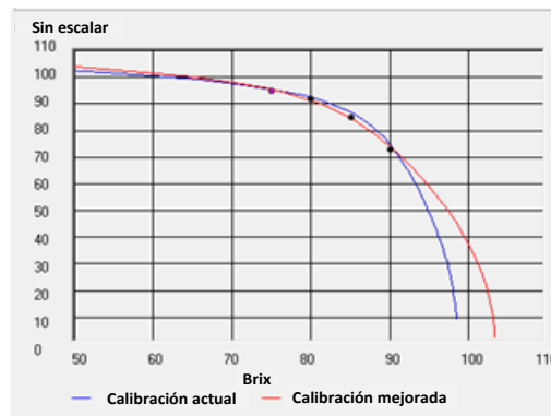
Ilustración 21: Ejemplo de una buena calibración de Brix
