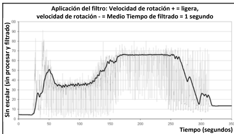
Ilustración 7: Filtrado de la señal sin escalar/sin procesar (1)
