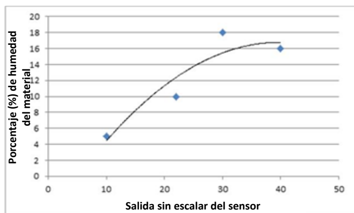
Ilustración 20: Ejemplo de una mala calibración cuadrática
