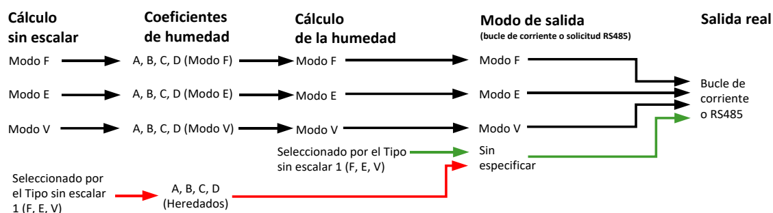
Ilustración 12: Selección de salida antigua
