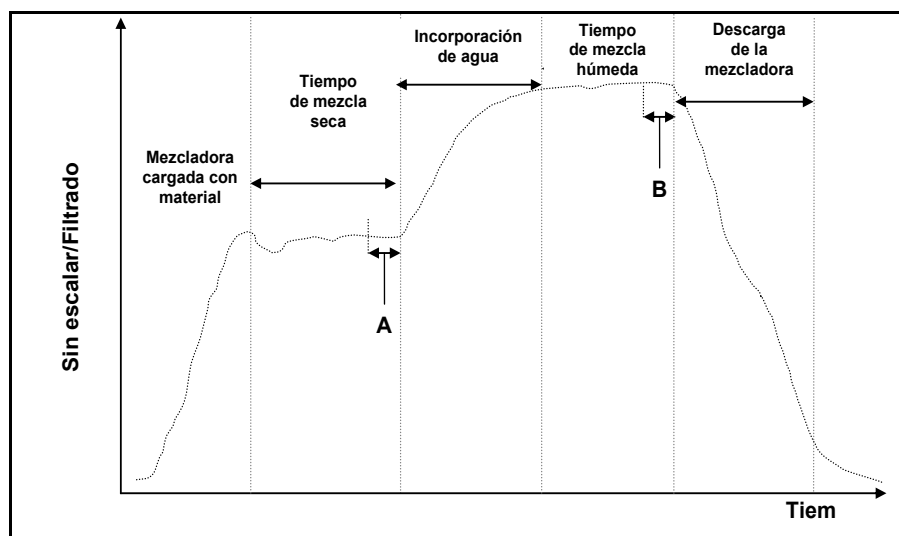
Ilustración 5: Curva de humedad normal
