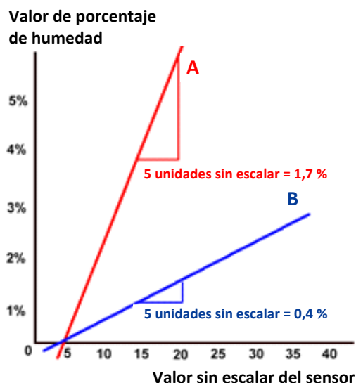
Ilustración 9: Relación de los valores Sin escalar respecto a la humedad
