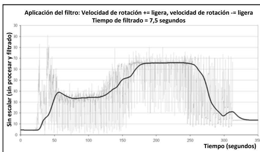
Ilustración 8: Filtrado de la señal SIN PROCESAR (2)
