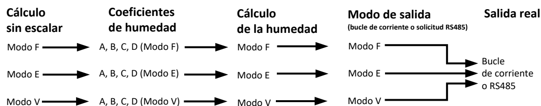
Ilustración 10: Disposición de los datos en el sensor
