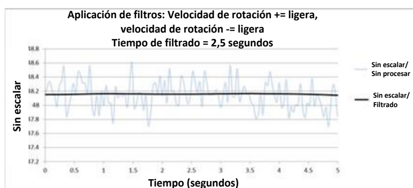
Ilustración 4: Gráfico que muestra la señal filtrada
