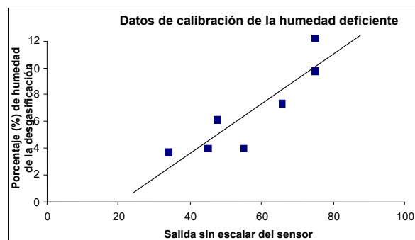
Ilustración 18: Ejemplos de malos puntos de calibración del material
