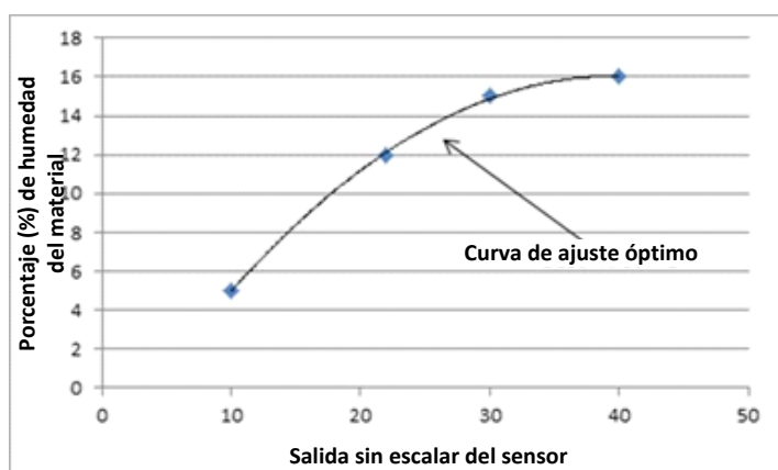
Ilustración 19: Ejemplo de una buena calibración cuadrática
