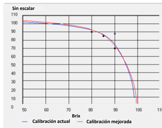
Ilustración 22: Ejemplo de una mala calibración de Brix
