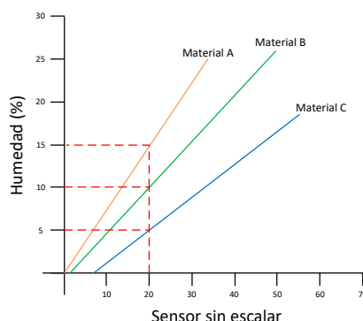
Ilustración 13: Calibraciones para 3 materiales diferentes
