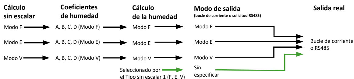
Ilustración 11: Ninguna selección de salida especificada
