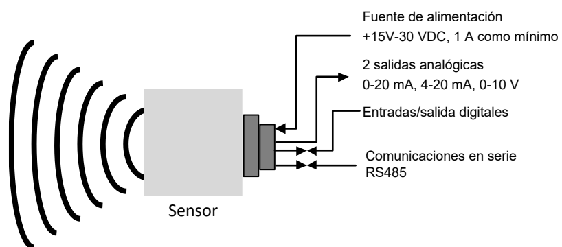
Ilustración 1: Conexión del sensor (descripción general)
