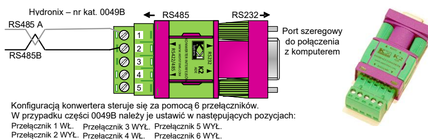
Rysunek 11: Połączenia konwertera RS232/485 (0049B)
