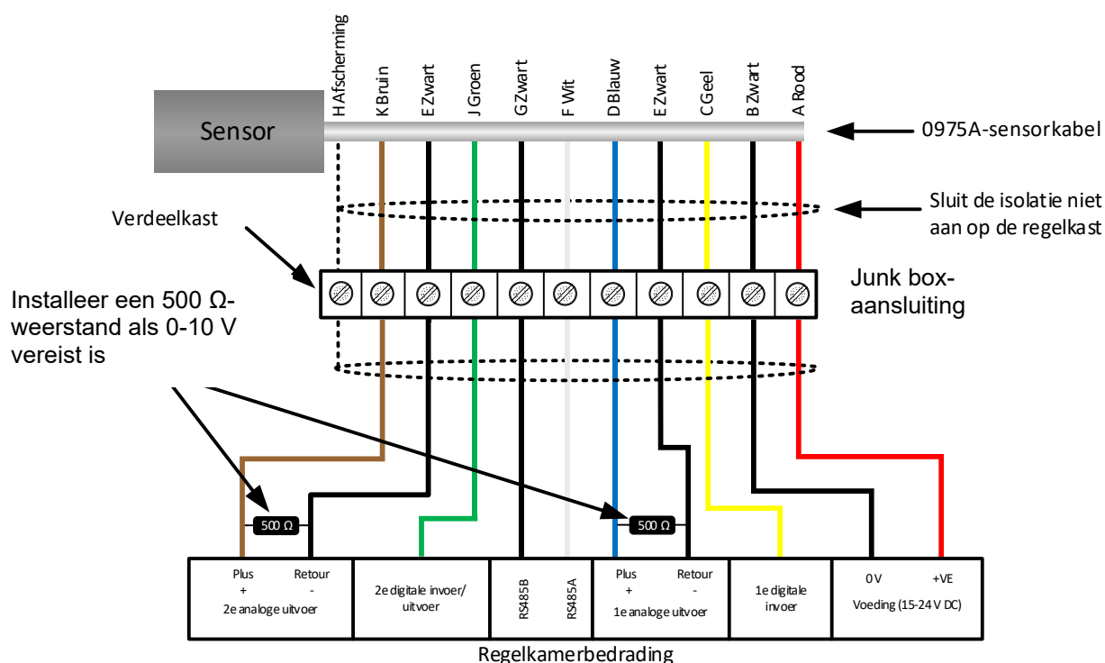
Afbeelding 1: 0975A-sensorkabelaansluitingen
