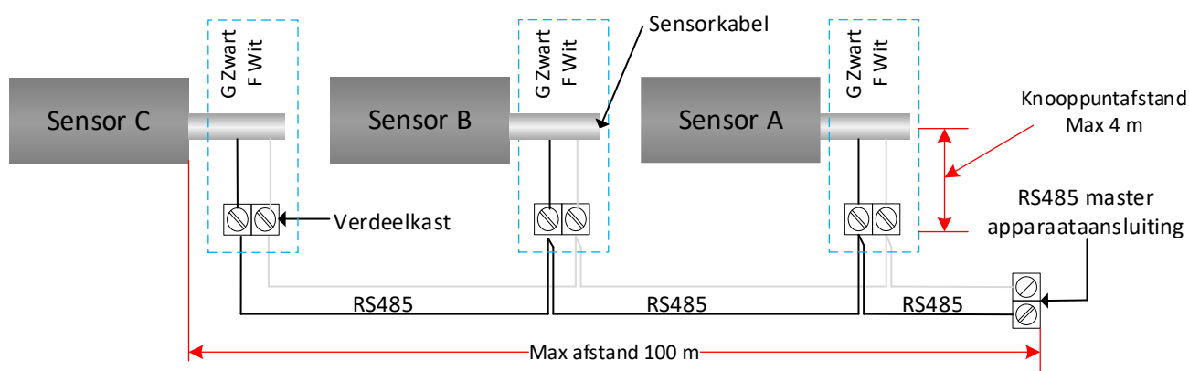
Afbeelding 2: RS485 Multidrop-netwerktopologie
