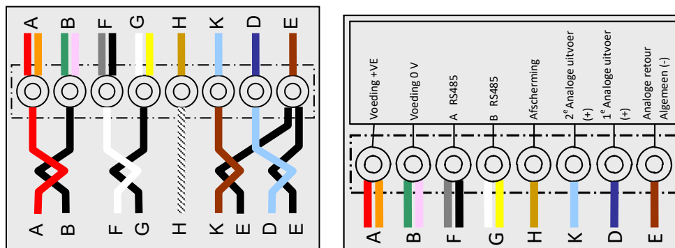
(A) Sensorkabelaansluitingen
