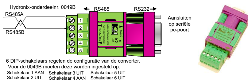
Afbeelding 11: RS232/485-converteraansluitingen (0049B)
