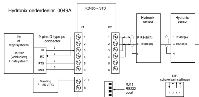
Afbeelding 12: RS232/485-converteraansluitingen (0049A)
