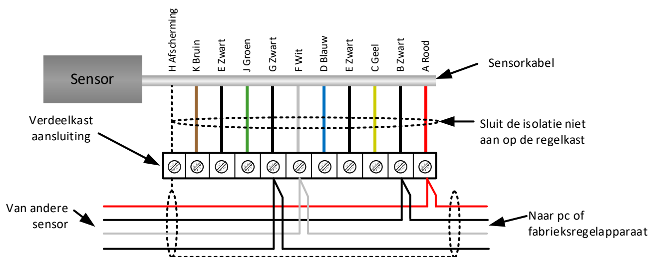
Afbeelding 3: RS485 Multidropaansluitingen
