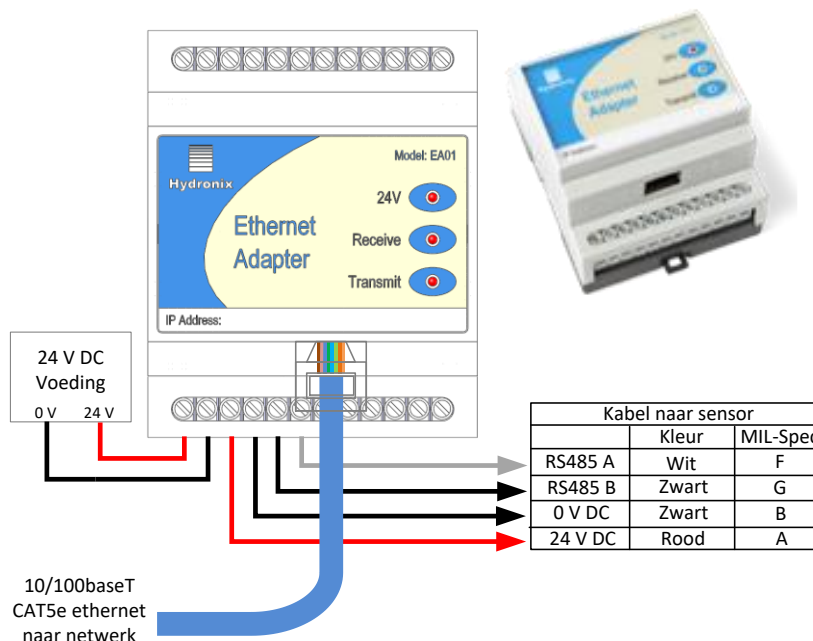
Afbeelding 14: ethernetadapteraansluitingen (EAK01)
