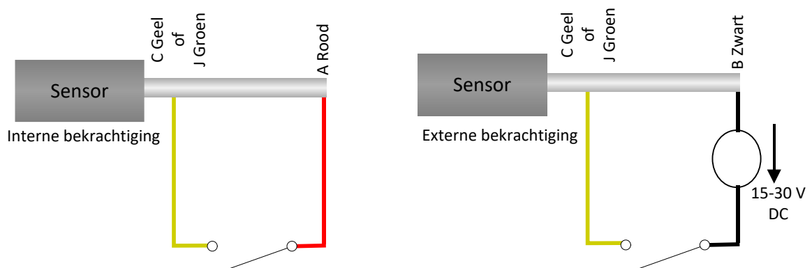
Afbeelding 6: interne/externe bekrachtiging van digitale invoer 1 en 2
