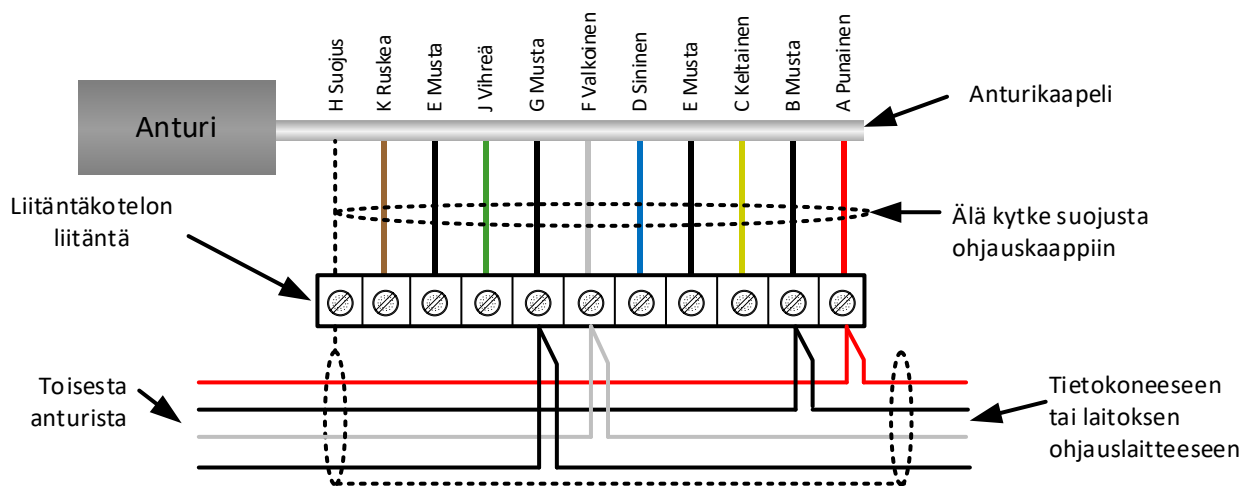
Kuva 3: RS485 monipisteliitännät
