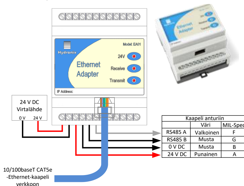
Kuva 14: Ethernet-sovitinliitännät (EAK01)
