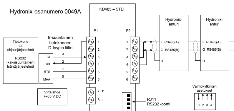
Kuva 12: RS232/485-muuntimen kytkennät (0049A)
