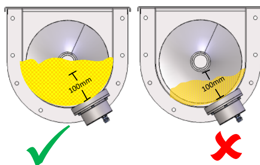
图7：螺旋输送机物料水平
