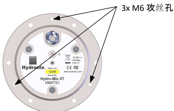
图16：攻丝孔
