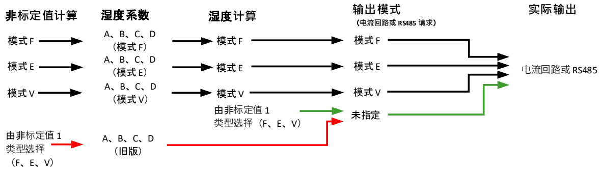
图 12: 旧输出选择
