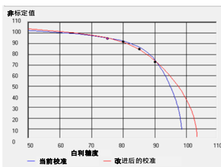
图 21: 良好白利糖度校准示例
