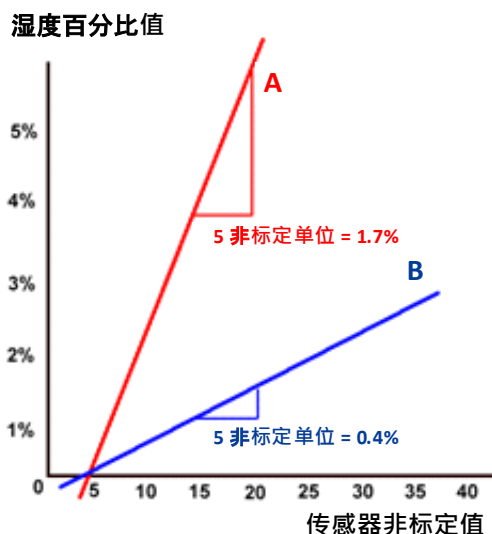
图 9：非标定值和湿度之间的关系
