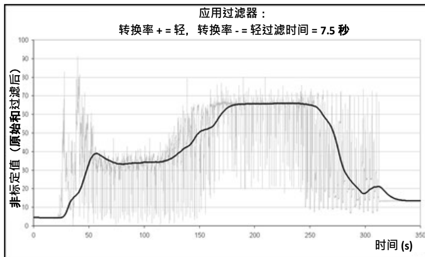
图 8：过滤原始信号（2）
