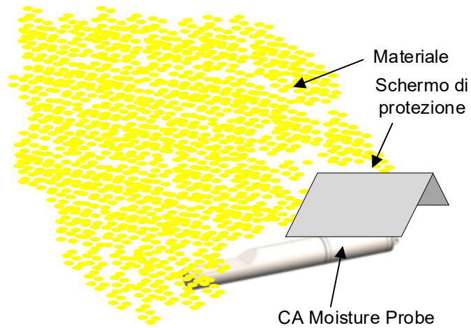
Figura 10. Schermo di protezione su CA Moisture Probe
