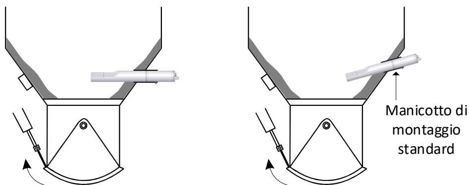
Figura 6. Montaggio di CA Moisture Probe sulla parete del contenitore
