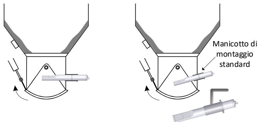
Figura 5. Montaggio di CA Moisture Probe sul collo del contenitore
