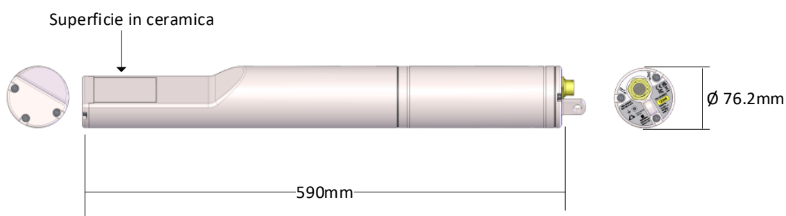
Figura 1. Il sensore CA Moisture Probe
