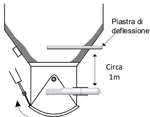
Figura 3. Installazione di una piastra di deflessione per prevenire danni
