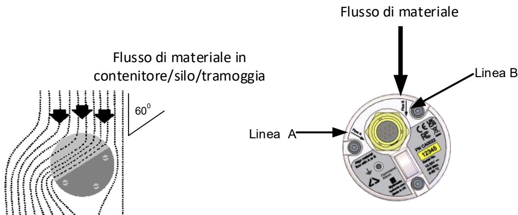
Figura 2. Angolo di montaggio di CA Moisture Probe XT e flusso di materiale
