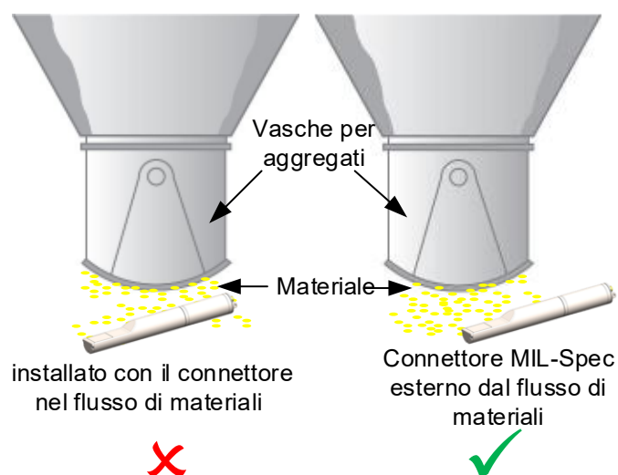
Figura 8. CA Moisture Probe installato sotto una vasca per aggregati
