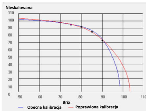
Rysunek 22: Przykład dobrej kalibracji do pomiaru stopnia Brix
