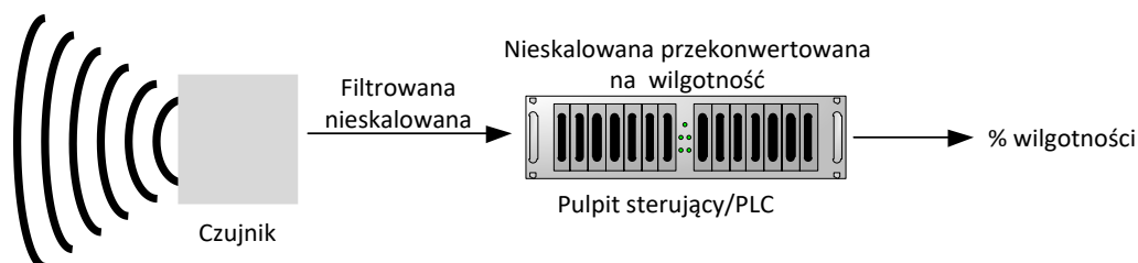
Rysunek 17: Kalibracja wewnątrz systemu sterowania
