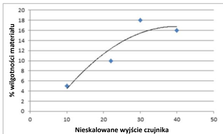
Rysunek 21: Przykład złej kalibracji kwadratowej
