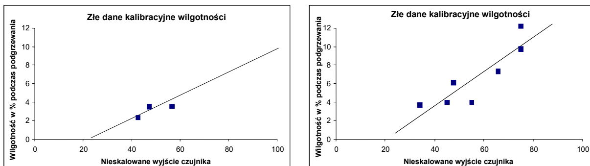
Rysunek 19: Przykłady nieprawidłowych punktów kalibracji względem materiału
