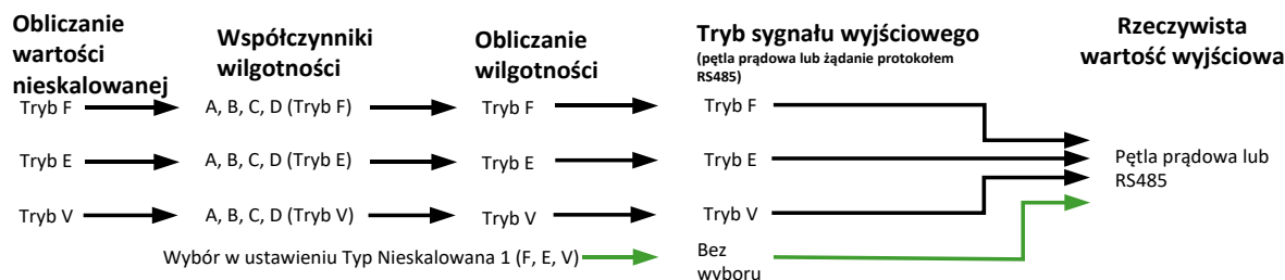
Rysunek 12: Bez wyboru konkretnego rodzaju sygnału wyjściowego
