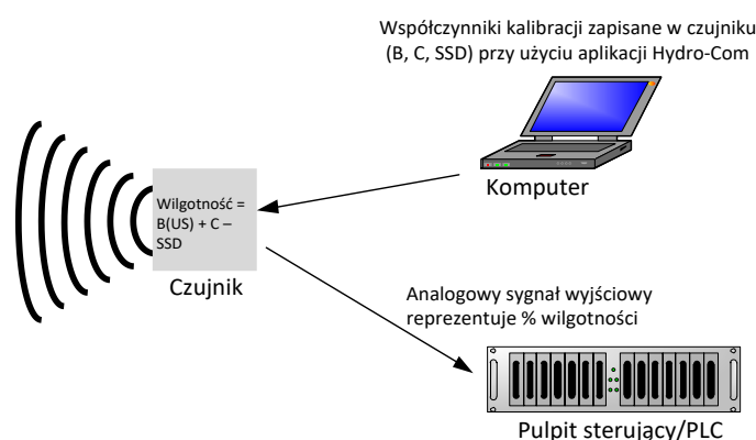
Rysunek 16: Kalibracja wewnątrz czujnika
