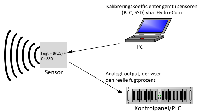
Fig. 16: Kalibrering i sensoren
