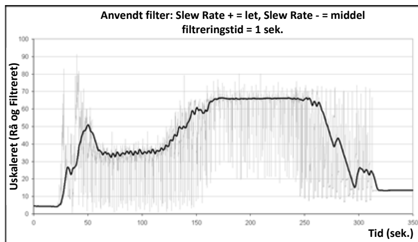
Fig. 8: Filtrering af Rå uskaleret-signal (1)
