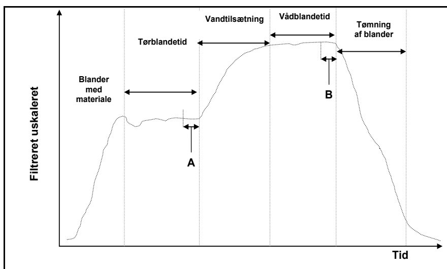
Fig. 6: Typisk fugtkurve
