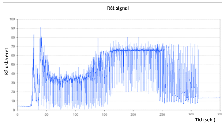
Fig. 7: Graf over det rå signal under en blandecyklus
