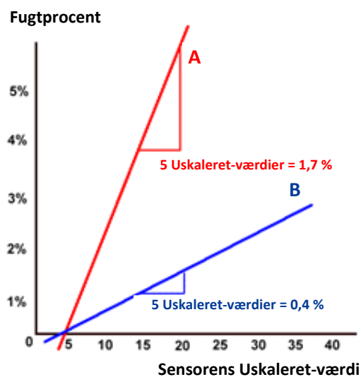
Fig. 10: Forhold mellem Uskaleret-værdi og Fugt
