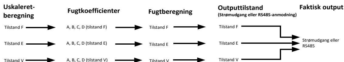
Fig. 11: Datasammensætning i sensoren
