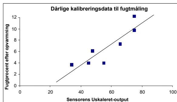
Fig. 19: Eksempler på dårlig materialekalibrering
