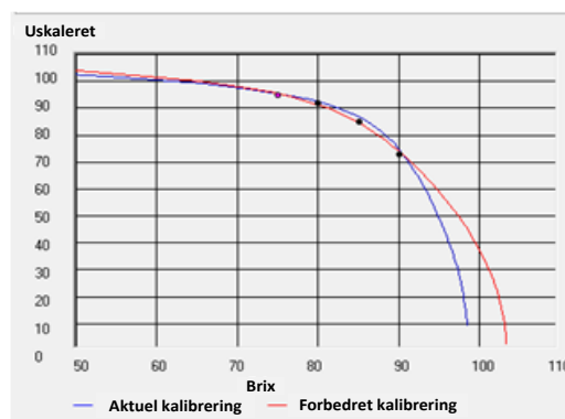
Fig. 22: Eksempel på god Brix-kalibrering
