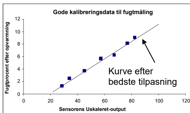
Fig. 18: Eksempel på god materialekalibrering
