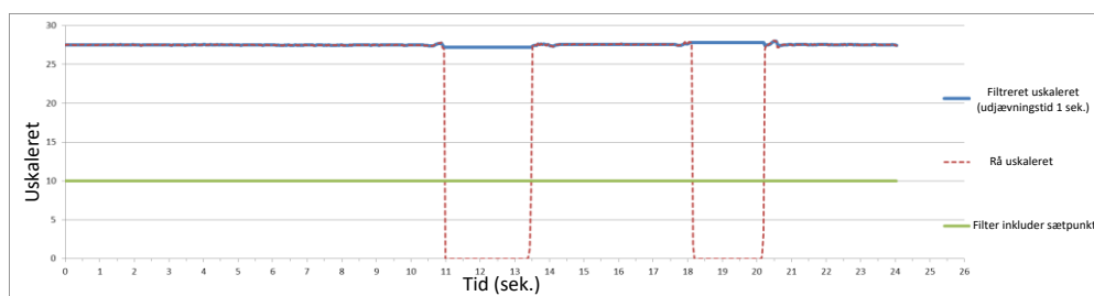
Fig. 3: Sensor-output med Rå og Filter inkluder
