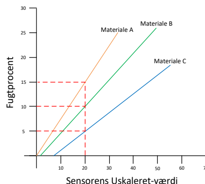
Fig. 14: Kalibreringer til tre forskellige materialer
