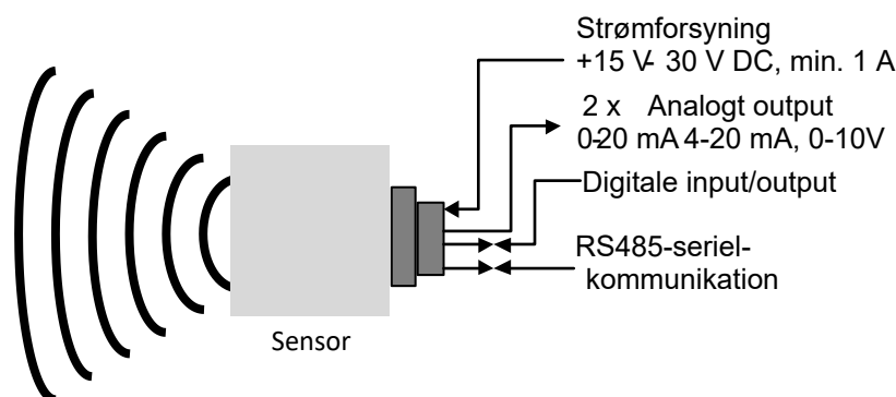
Fig. 1: Sensortilslutning (oversigt)
