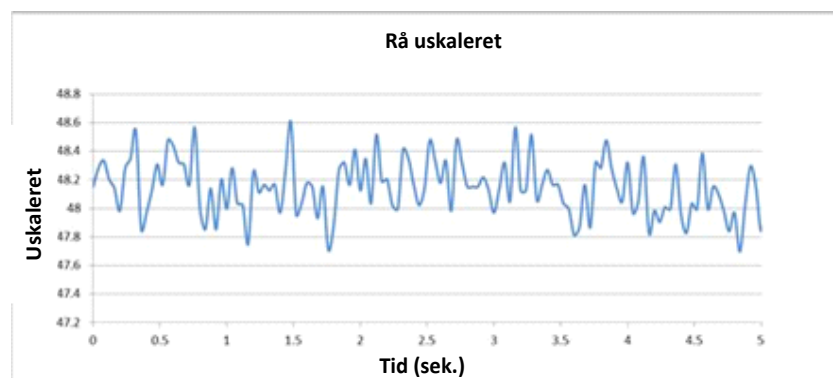
Fig. 4: Rå uskaleret-overvågning af fugtindhold i strømmende materiale
