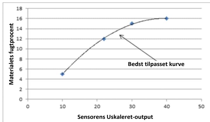
Fig. 20: Eksempel på god kvadratisk kalibrering
