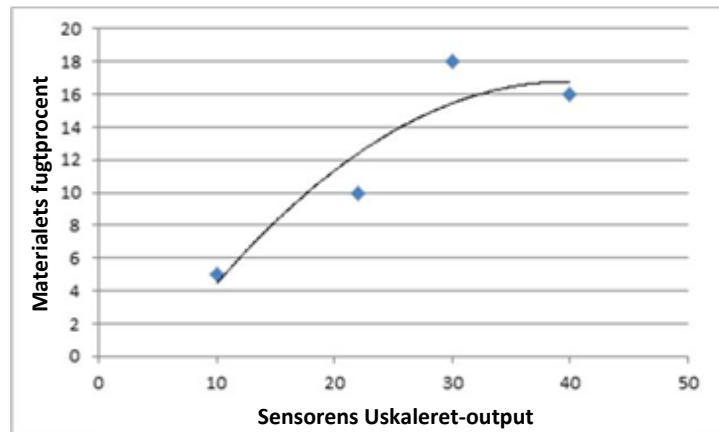
Fig. 21: Eksempel på dårlig kvadratisk kalibrering
