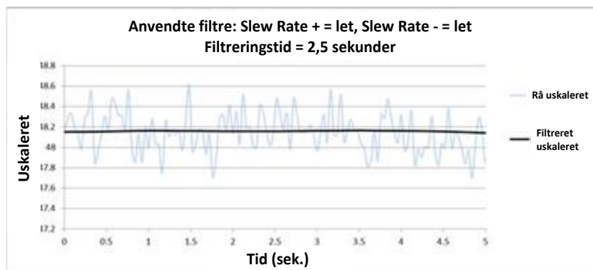
Fig. 5: Graf over det filtrerede signal
