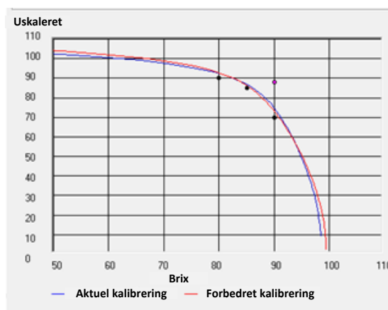
Fig. 23: Eksempel på dårlig Brix-kalibrering
