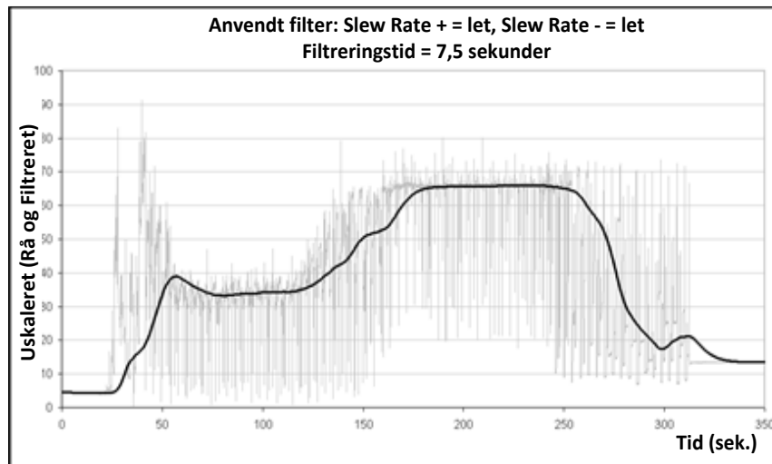
Fig. 9: Filtrering af rå signal (2)
