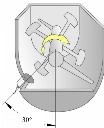
Imagem 6: Instalação do Misturador de Veio Simples
