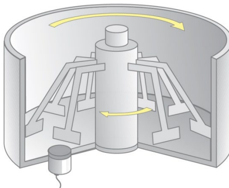
Imagem 4: Instalação do Misturador Turbo
