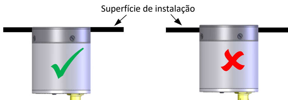
Imagem 2: Instalação em Superfície Plana
