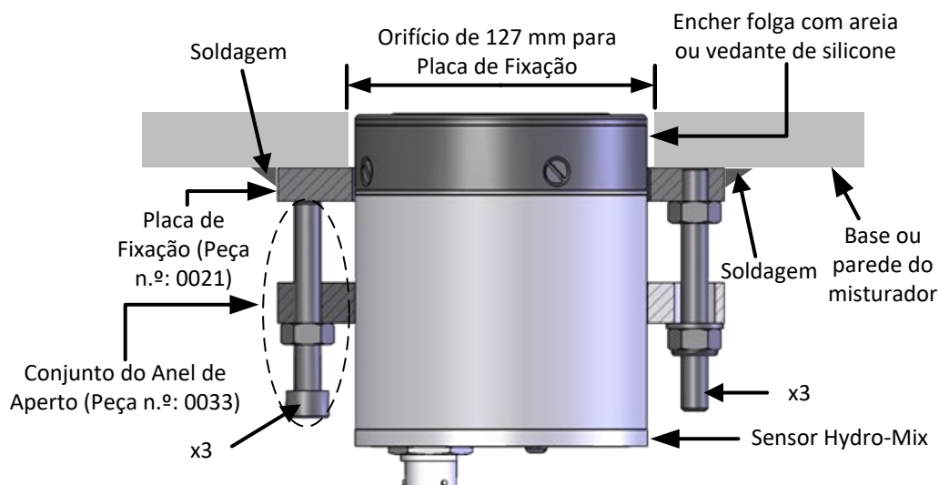
Imagem 11: Instalação do Sensor
