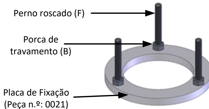
Imagem 13: Placa de Fixação Preparada para Instalação do Anel de Aperto
