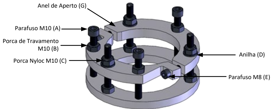
Imagem 14: Anel de Aperto Ajustável Montado e Instalado na Placa de Fixação
