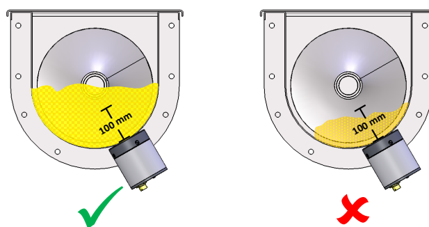
Imagem 9: Nível de Material do Transportador Helicoidal
