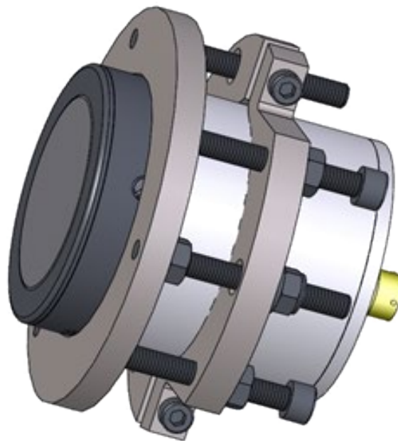
Imagem 15: Anel de Aperto Ajustável (0033) Instalado na Placa de Fixação (0021) e Hydro-Mix
