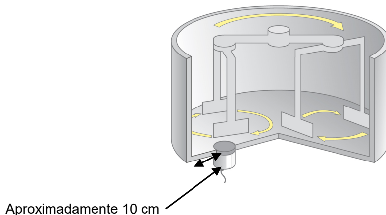
Imagem 5: Instalação do Misturador Planetário
