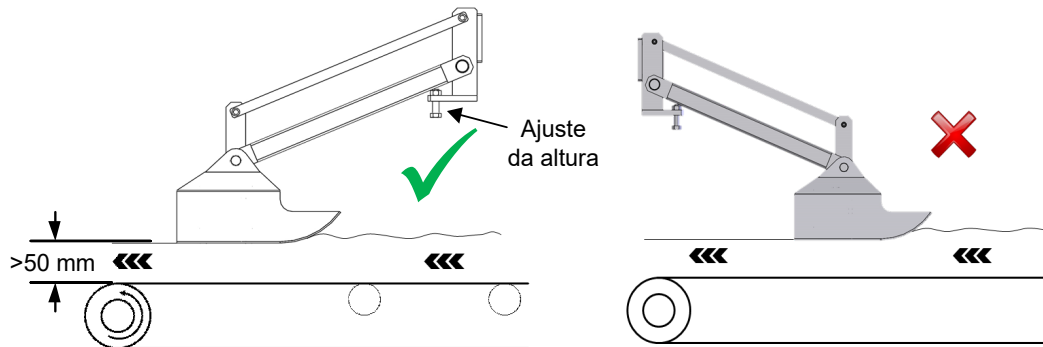
Imagem 10: Instalação do Hydro-Skid numa Correia Transportadora
