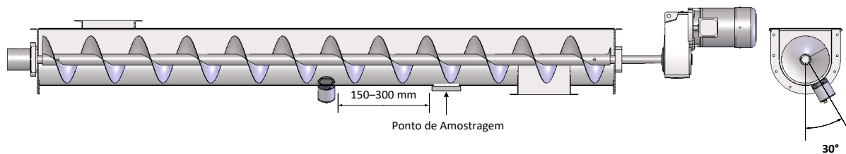
Imagem 8: Instalação do Transportador Helicoidal
