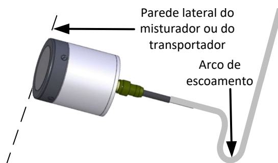
Imagem 17: Hydro-Mix Instalado com um Arco de Escoamento
