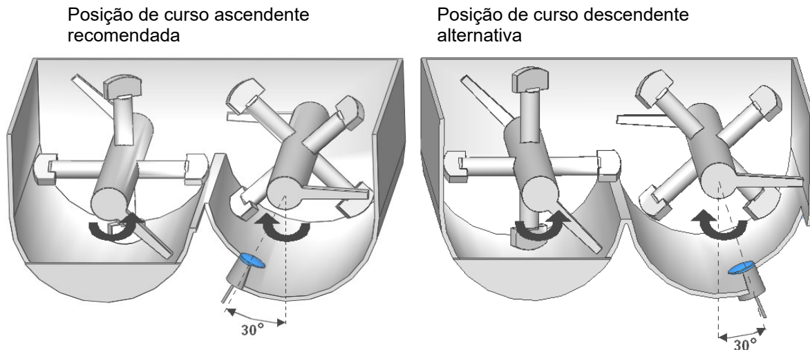
Imagem 7: Instalação do Misturador de Veio Duplo
